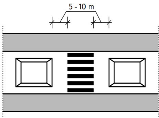
Фиг. 4а. Разположение на пътни възглавници спрямо пешеходна пътека
