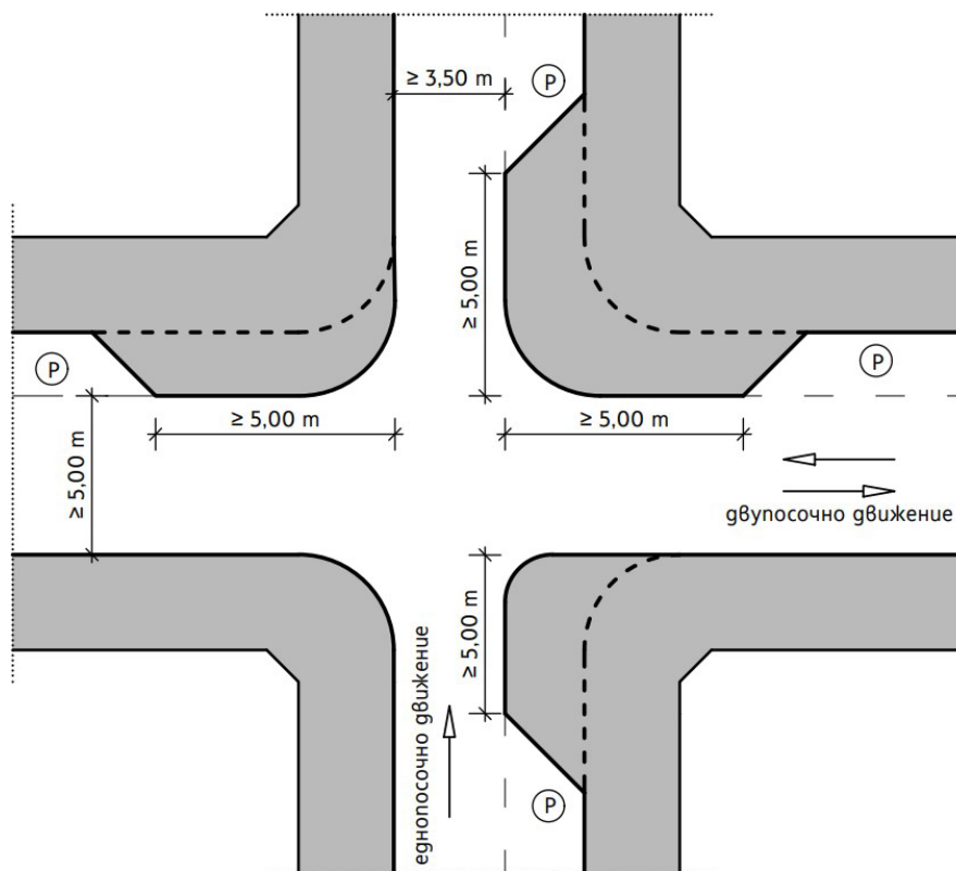
Фиг. 12. Схема на изнесени тротоари в кръстовище
