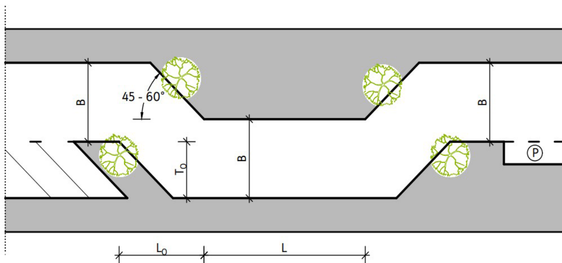
Фиг. 6б. Шикан
