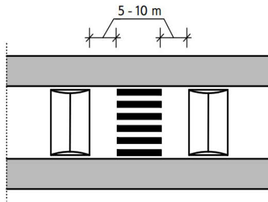
Фиг. 4б. Разположение на гърбици спрямо пешеходна пътека
