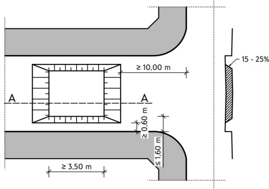
Фиг. 2б. План и напречен разрез на пътна възглавница
