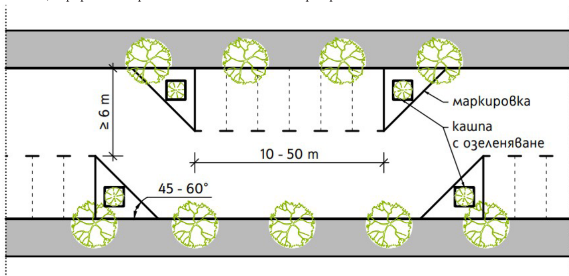
б) шикан, оформен с преместваеми кашпи, маркировка и реорганизация на паркирането 6507
