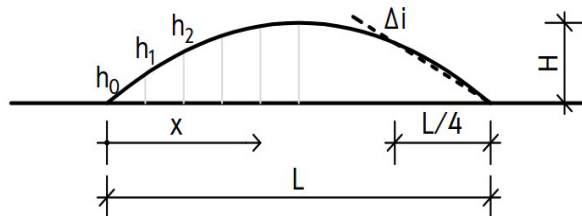
Фиг. 1. Параболично сечение на гърбица
