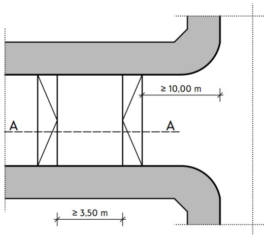
Фиг. 2а. План на пътна табла
