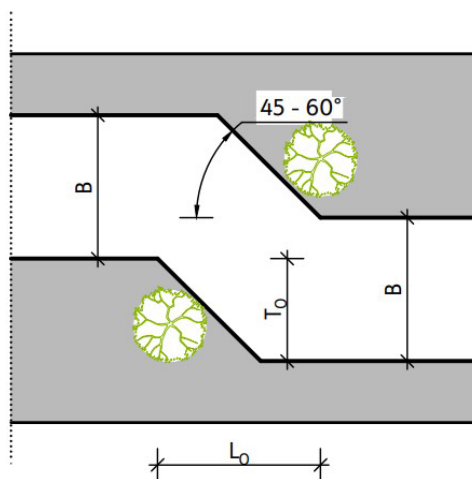
Фиг. 6а. Хоризонтално отместване
