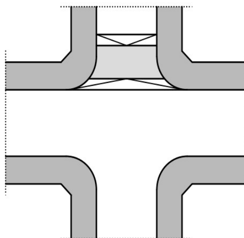
Фиг. 4г. Повдигане продължението на тротоарите в зоната на кръстовище чрез пътна табла
