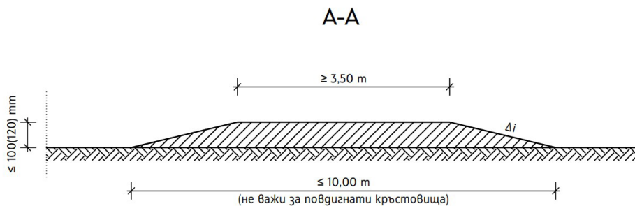
Фиг. 2г. Надлъжен разрез на пътна табла, на пътна възглавница и на повдигнато кръстовище
