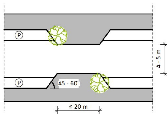
Фиг. 10б. Двустранно локално стеснение
