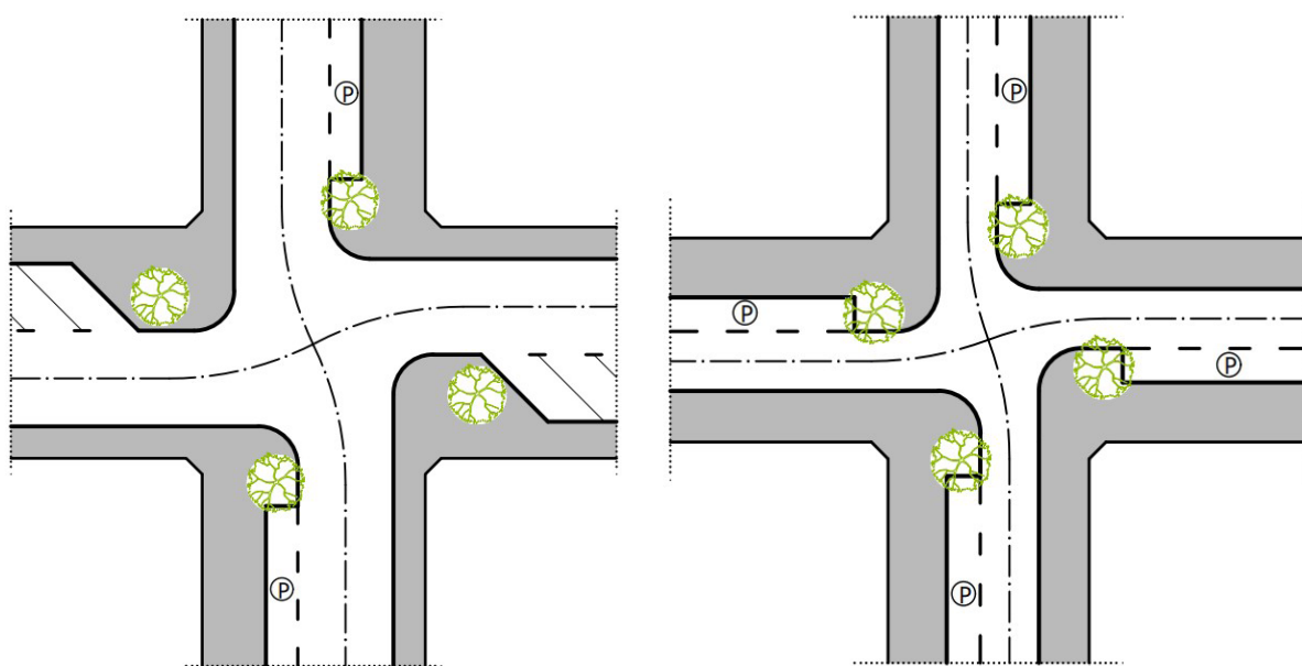
Фиг. 9а. При улици с габарит, по-голям от 12 m и двупосочно движение
