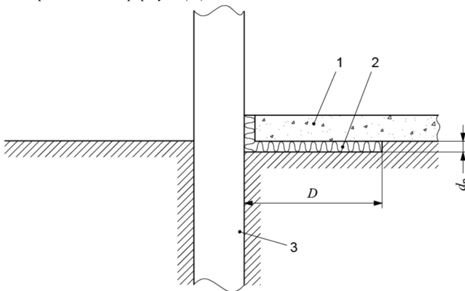
Фигура 4. Принципна схема на хоризонтална топлоизолация по периферията
