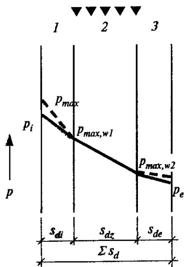
Фиг. 2.5а. Дифузия на водната пара с кондензационен пад във вътрешността на ограждащата конструкция или елемент
