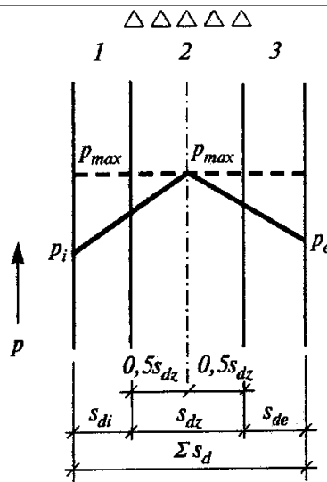
Фиг. 2.5б. Дифузия на водната пара по време на изпаряването след кондензационен пад във вътрешността на ограждащата конструкция или елемент
