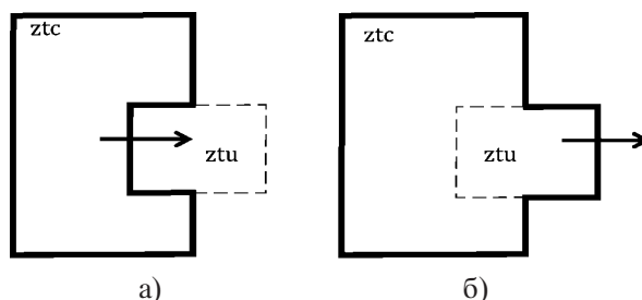
Фигура 1. Външна и вътрешна топлинно неклиматизирана зона: а) външна топлинно неклиматизирана зона (z tu ); б) вътрешна топлинно неклиматизирана зона (z tu )
