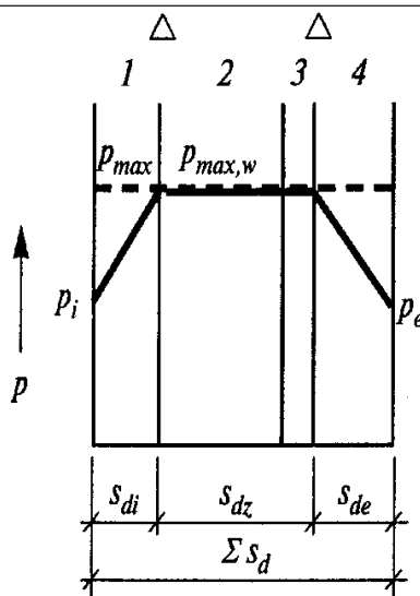
Фиг. 2.4б. Дифузия на водната пара по време на изпарението след кондензационен пад в две равнини на ограждащата конструкция или елемент
