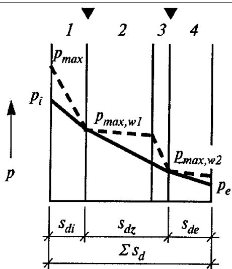
Фиг. 2.4а. Дифузия на водната пара с кондензационен пад в две равнини на ограждащата конструкция или елемент (между слоеве 1 и 2 и между слоеве 3 и 4)
